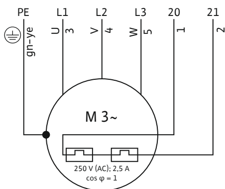
Fig. 8: Anschlussplan 3~Motor
