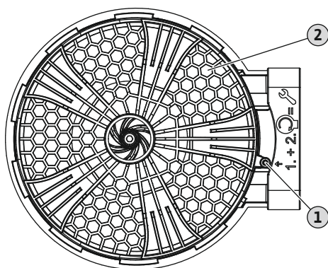
Fig. 9: Bodenplatte abbauen
