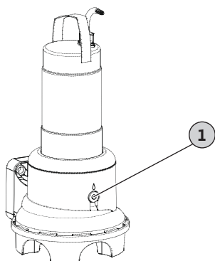
Fig. 10: Dichtungskammer: Ölwechsel
