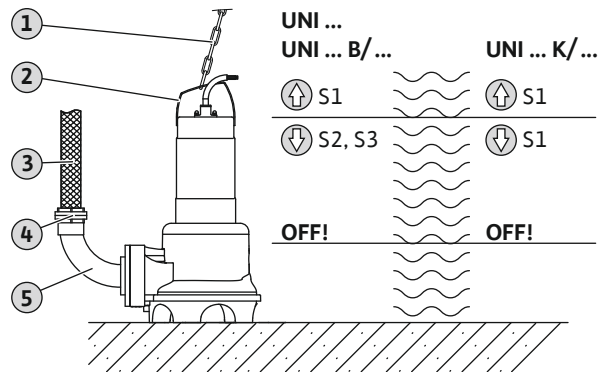
Fig. 6: Nassaufstellung, transportabel
