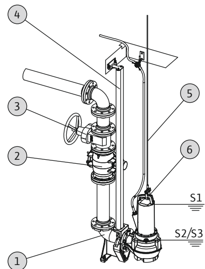
Fig. 5: Nassaufstellung, stationär
