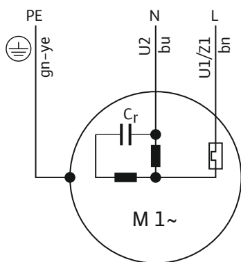
Fig. 7: Anschlussplan 1~Motor
