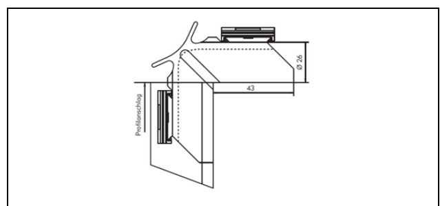
Abb. 5: Maßzeichnung HZ-Außeneckschelle
