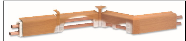
Abb. 1: HZ-Ecklösungen
