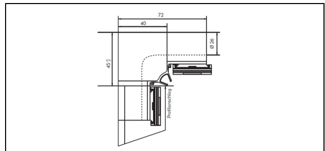
Abb. 3: Maßzeichnung HZ-Inneneckschelle
