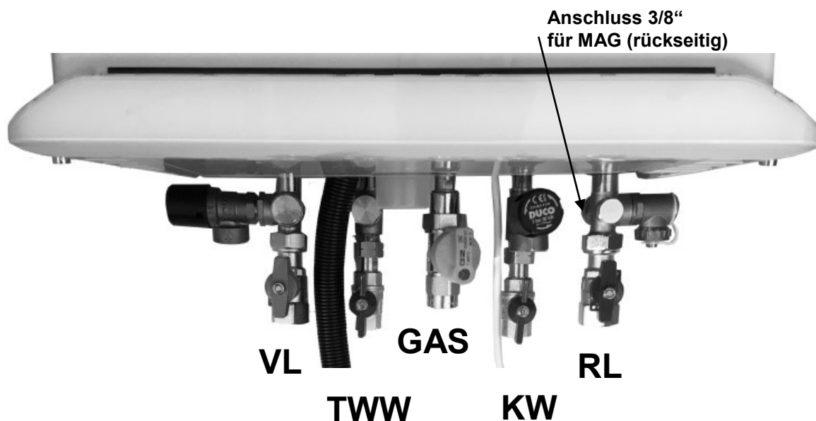
Abb. 2: Hydraulische Trinkwasseranschlüsse inkl. einem zusätzlichen Sicherheitsventil von max. 8 bar
