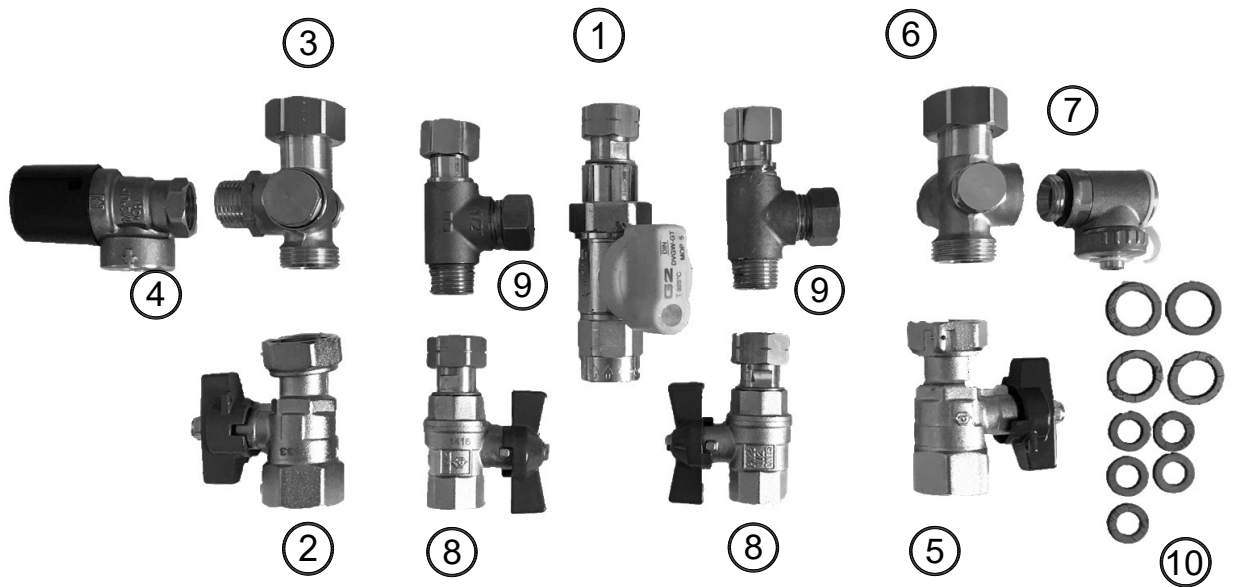
Abb./Fig. 1: Lieferumfang Anschluss-Set Kombi 96.33000-7226
