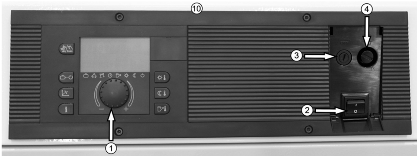
Abb. 79: Kesselschaltfeld
