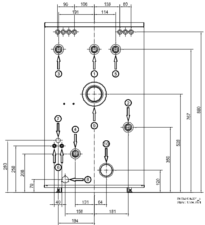
Abb. 3: Abmessungen Rückseite
