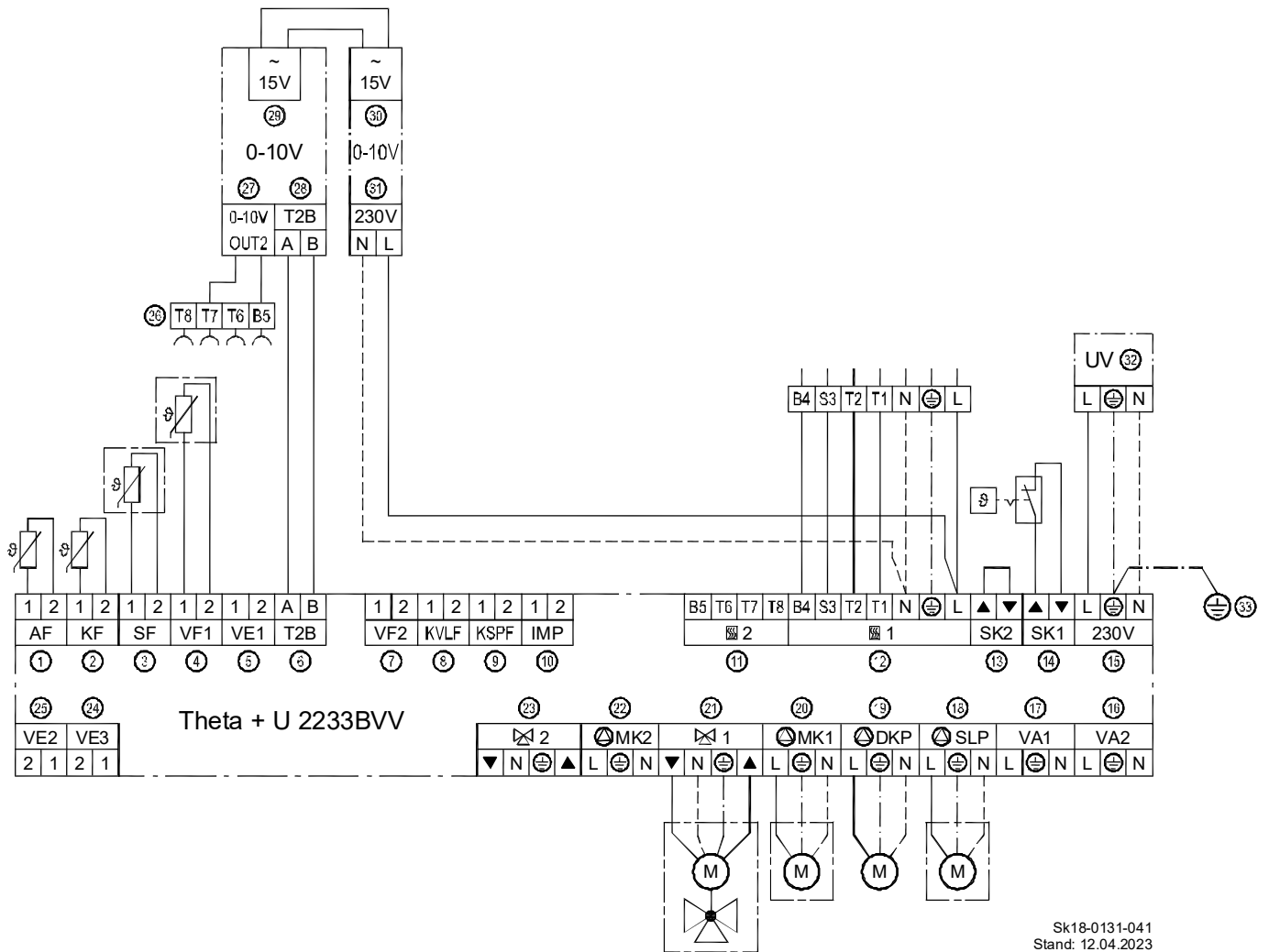
Abb. 25: Elektrische Anschlüsse und Stromlaufplan für ecoDUO...m (Raket Brenner® RM .. EUG)
