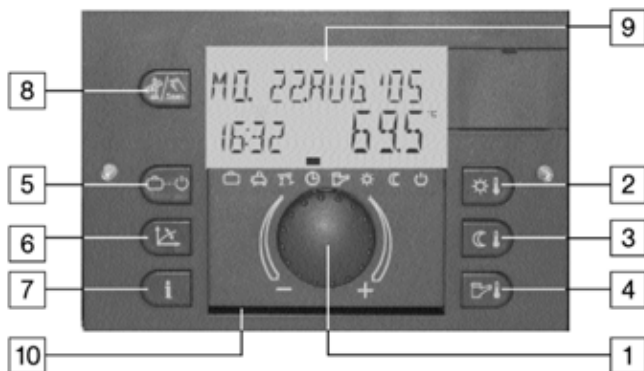
Abb. 56: Bedieneinheit
