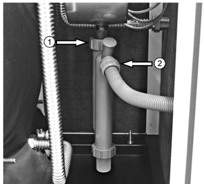
Abb. 67: Demontage des Kondensat-Siphons
