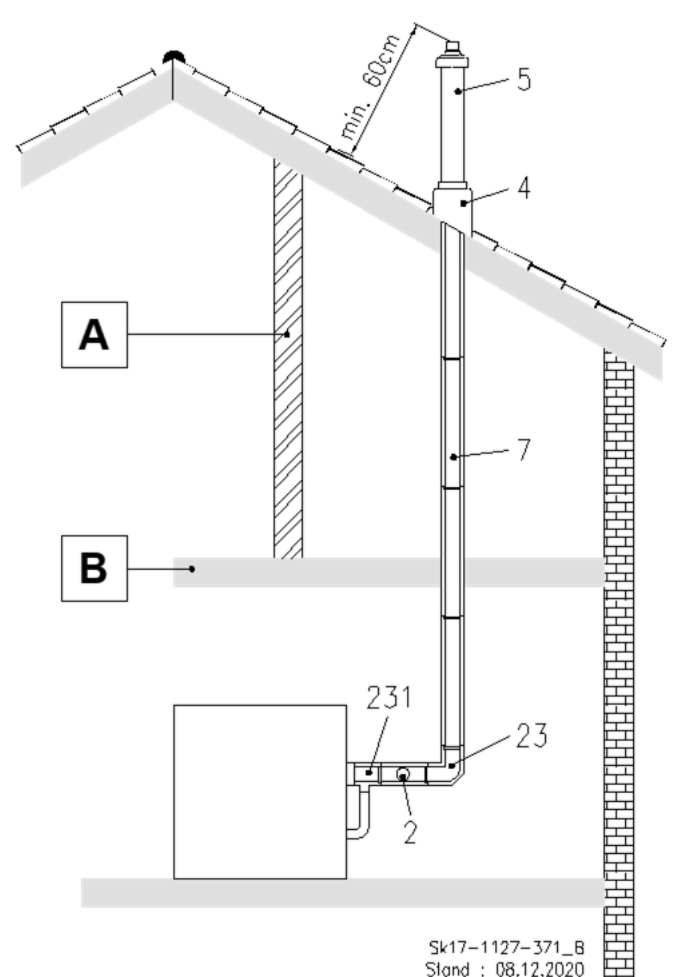
Abb. 32: C 33x Luft-Abgas-Rohrsystem senkrecht durch eine Decke und eine Dachhaut
