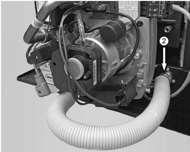
Abb. 63: Brenner-Gasanschluss ② am Kessel
