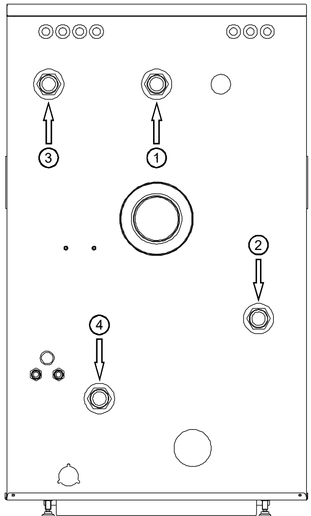
Abb. 13: Hydraulische Anschlüsse an der Kesselrückwand
