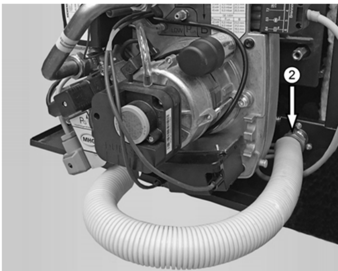
Abb. 12: Brenner-Gasanschluss ② am Kessel
