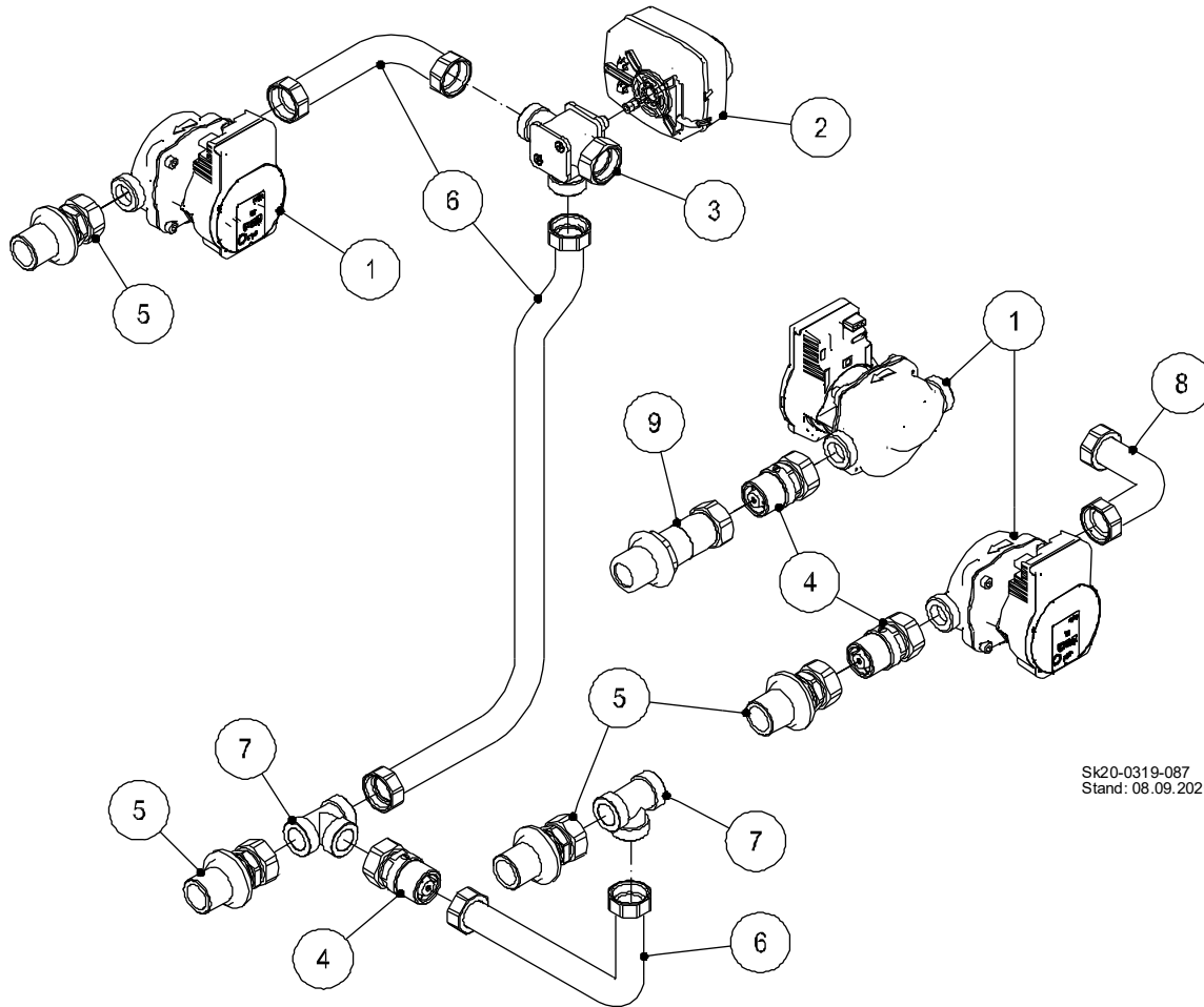
Abb. 77: Pumpen-, Mischerkreis und Speicherladeset
