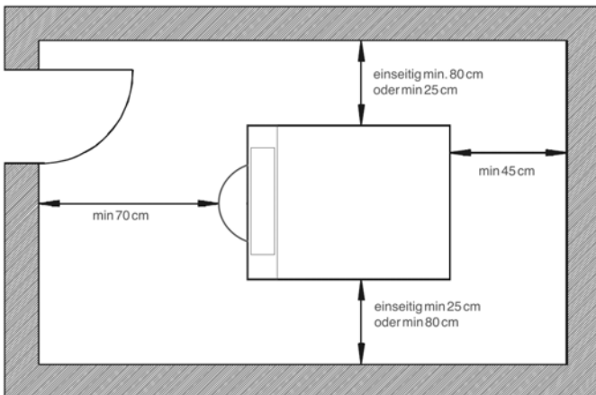
Abb. 1: Empfohlene Wandabstände
