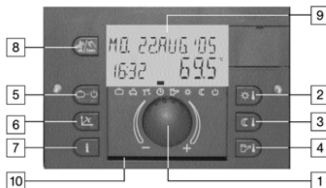
Abb. 74: Bedieneinheit
