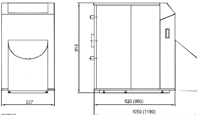
Abb. 2: Abmessungen
