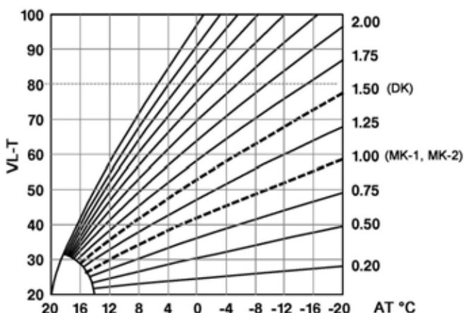
Abb. 57: Heizkennlinie (Steilheit)
