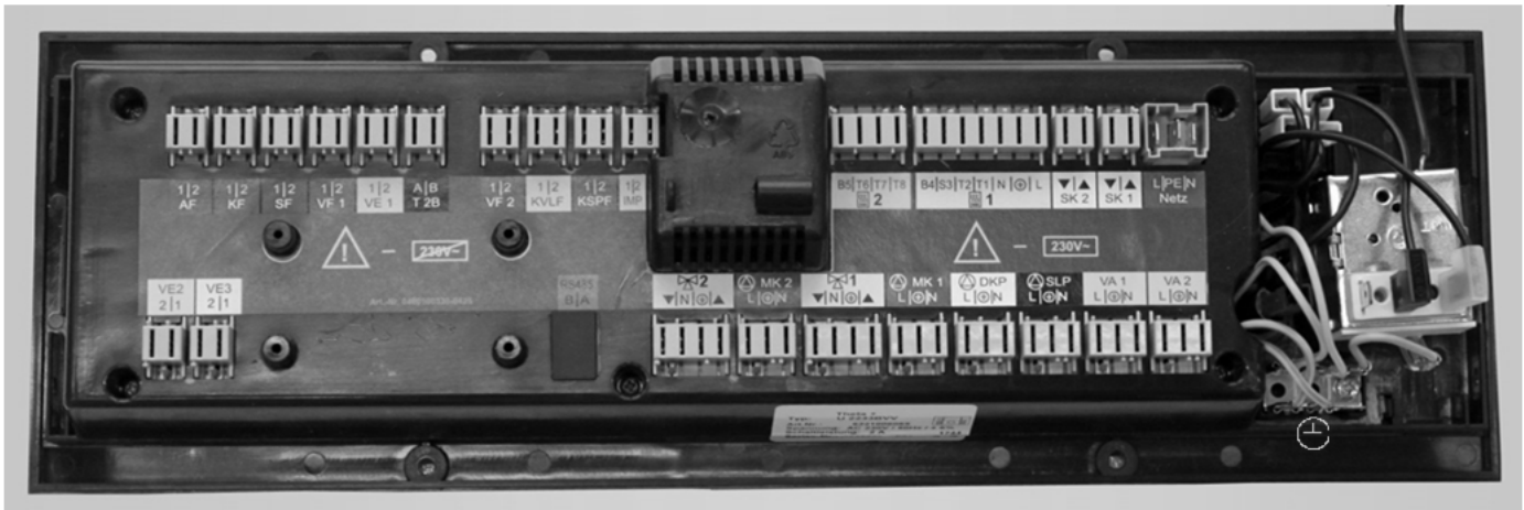
Abb. 24: Rückseite des Unit-Schaltfeldes
