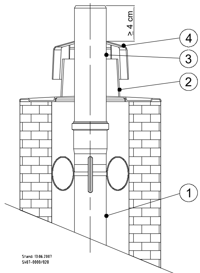
Abb. 43: Schachtabdeckung
