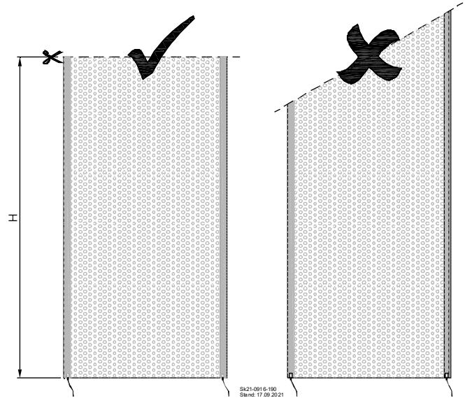
Abb. 3: Filmzuschnitt
