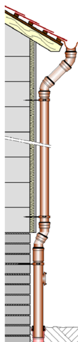
LORO-X Regenstandrohr aus Kupfer mit LORO-N Bogen mit LORO-X Sprungrohr bei Fassadenversprung
