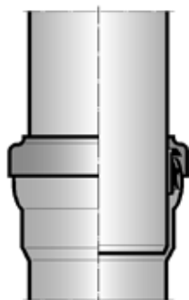
LORO-X Regenstandrohrkappe für herkömmliche Regenfalleitungen oder LORO-X Regenfalleitungen mit Aussendurchmesser 102 mm (mit Dichtelement)
