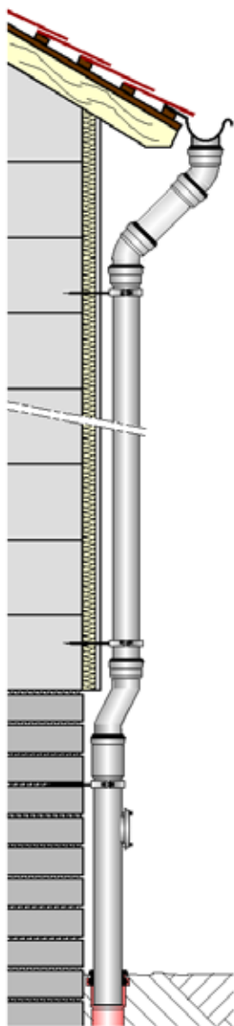
Installation an der Fassade mit LORO-X Regenstand- und Regenfallrohren
