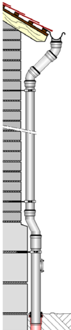
LORO-X Regenstandrohr aus Stahl, mit LORO-X Sprungrohr bei Fassadenversprung
