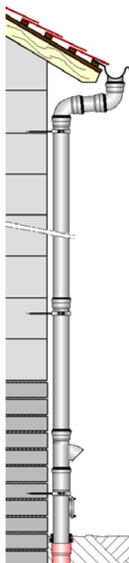
LORO-X Regenstandrohr mit Laubfang-Formteil
