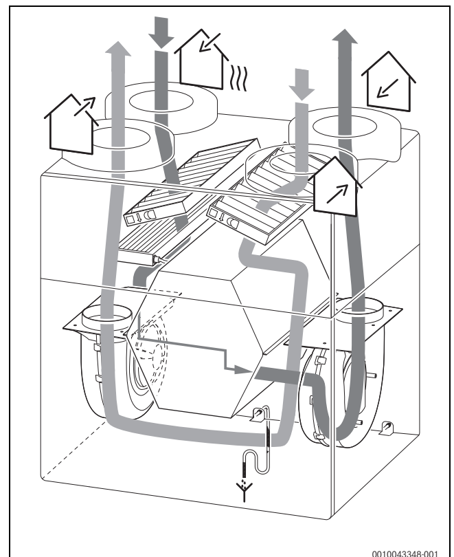
Bild 10 Beispiel Luftführung Bypassbetrieb bei Variante B
