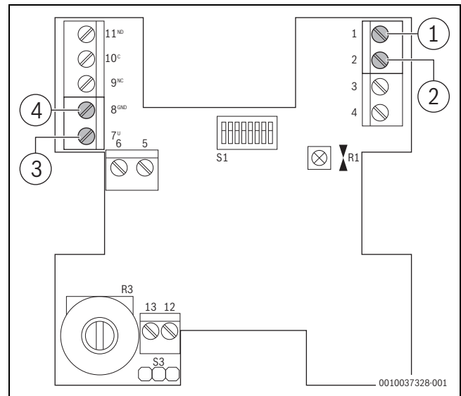
Bild 54 Interne elektrische Anschlüsse CS/VS-R
