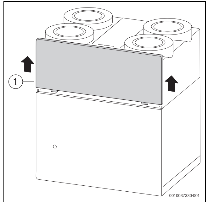
Bild 22 Abdeckblende Filter (Metall) abnehmen
