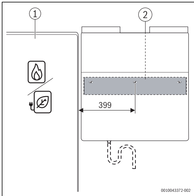
Bild 34 Abstand Bosch Wärmegerzeuger zu V5001C...
