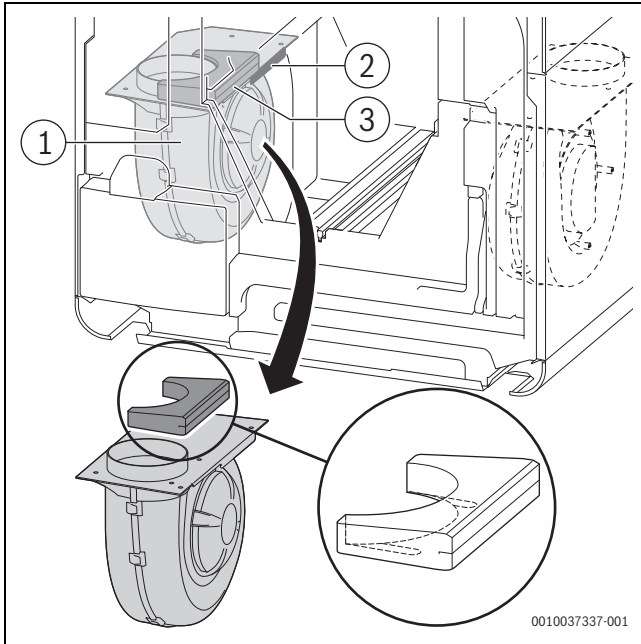
Bild 62 Gebläse herausziehen
