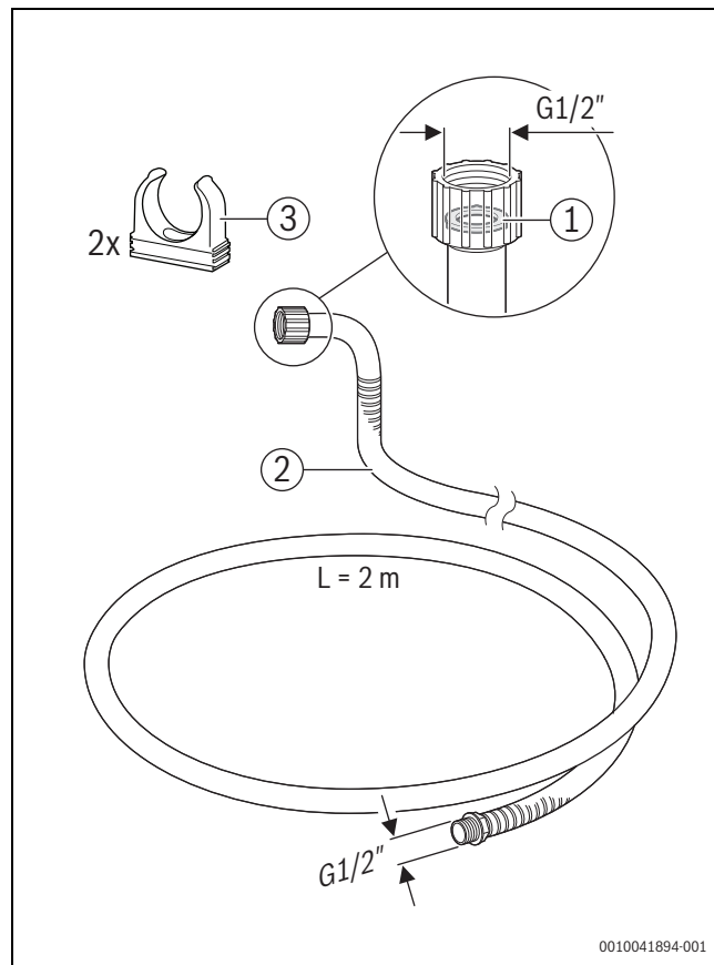
Bild 37 Schlauchsiphon-Anschluss-Set
