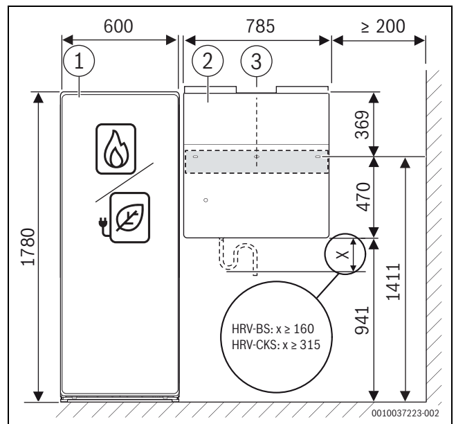
Bild 33 Einbaumaße im System mit einem Bosch Wärmerezeuger
