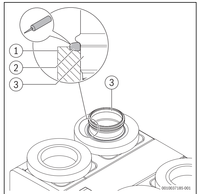
Bild 43 Doppelnippel FM160 abdichten
