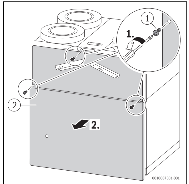
Bild 23 Schrauben lösen und Abdeckblende des EPP-Grundkörpers (Metall) abnehmen
