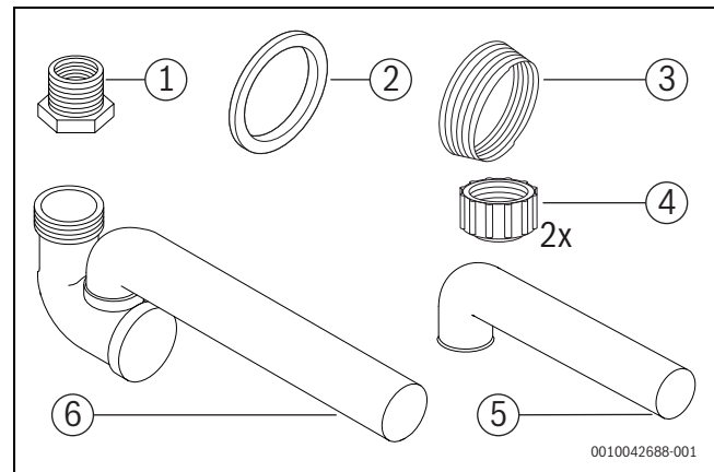
Bild 39 Kugelsiphon-Anschluss-Set
