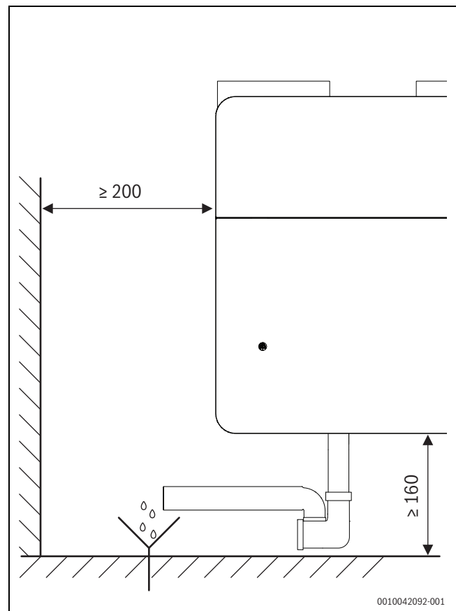
Bild 40 Mindestabstände V5001C... mit Siphon HRV-BS
