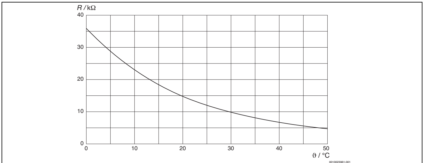
Bild 69 Kennlinie TV1 (12K)
