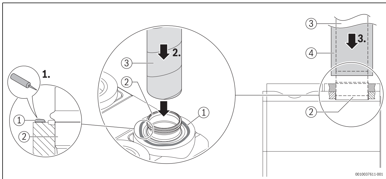
Bild 44 Aufbau Luftrohranschluss
