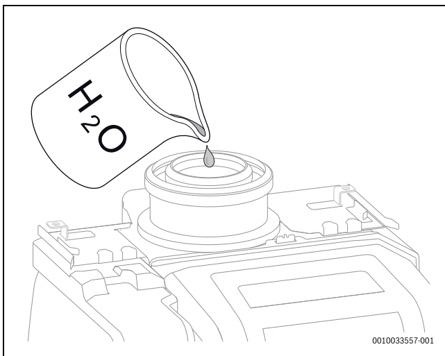
Bild 45 Kondensatsiphon mit Wasser füllen
