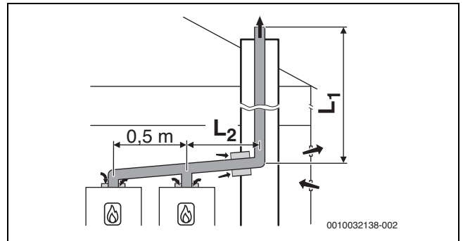
Bild 32 Kaskade mit 2 Geräten: Starre Abgasführung im Schacht nach B 53P mit raumluftabhängiger Luftzufuhr am Gerät
