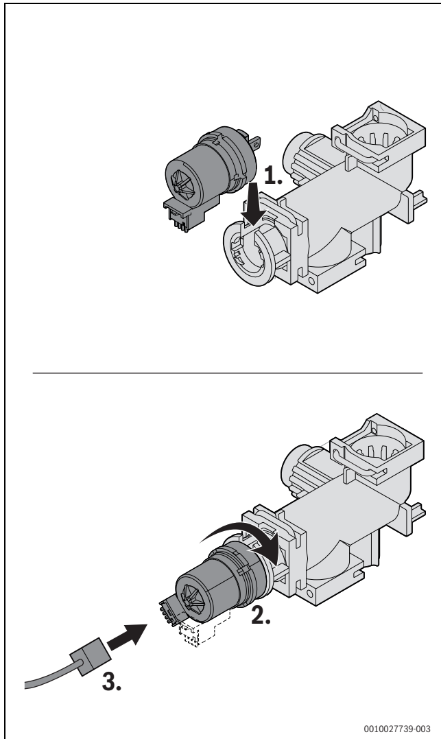
Bild 92 Motor einbauen (Variante ohne Schrauben)
