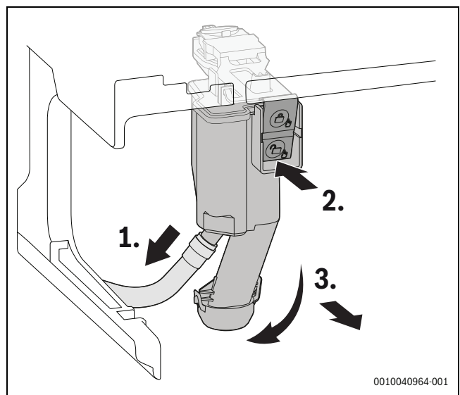
Bild 80 Kondensatsiphon ausbauen
