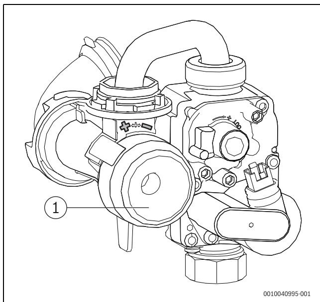
Bild 67 Gas-Luft-Verhältnis einstellen
