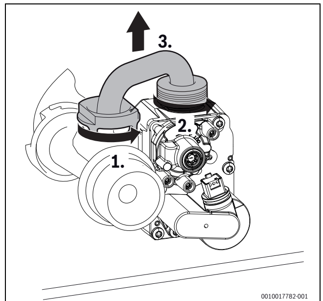
Bild 84 Gasrohr ausbauen
