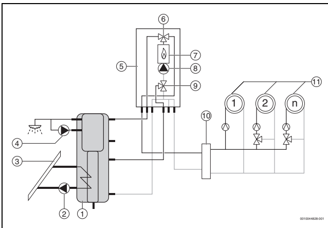
Bild 7 Condens 9800i WA mit Kombispeicher und Solarthermie mit drei Anschlussleitungen
