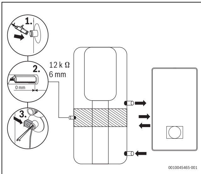
Bild 54 Pufferspeicher-Temperaturfühler 7735502289 einsetzen (bei Kombispeicher)
