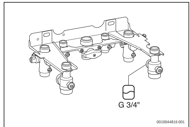
Bild 37 Ausdehnungsgefäß anschließen
