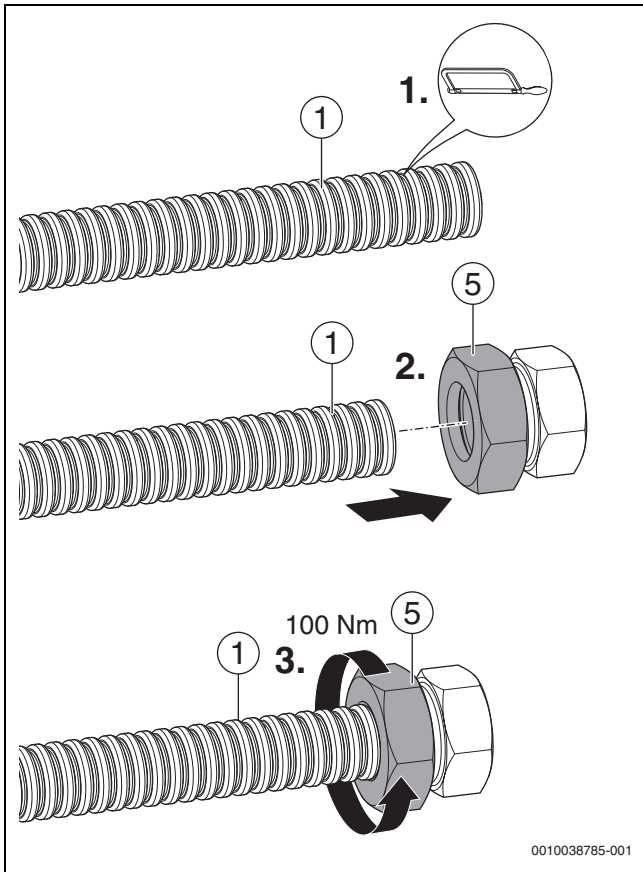
Bild 50 Verbindungsleitungen auf die korrekte Länge kürzen und Überwurfmutter anbringen
