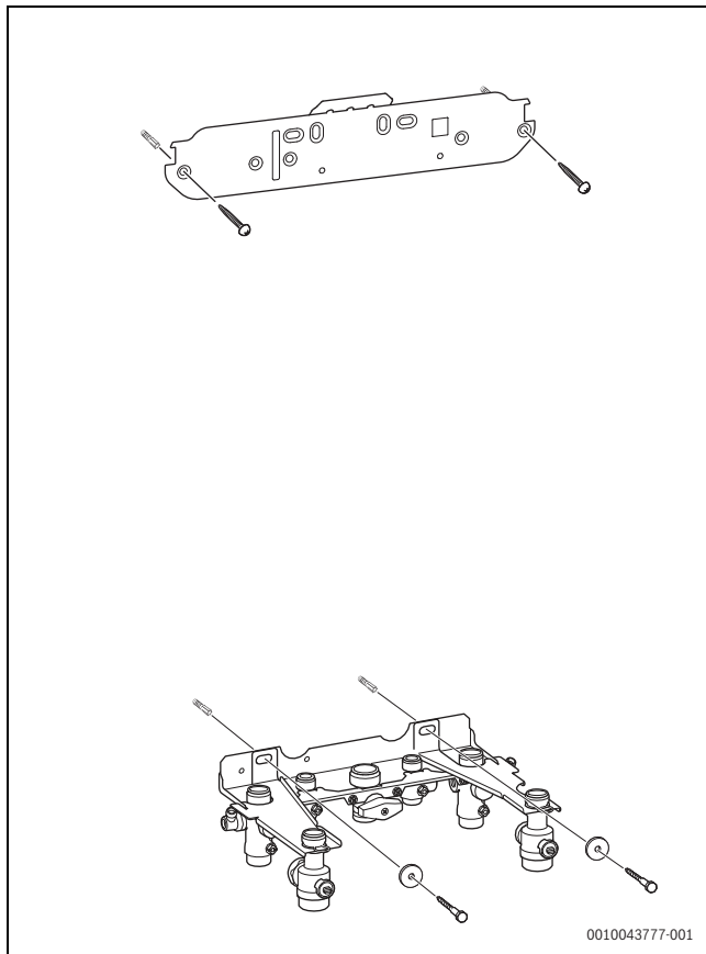
Bild 38 Befestigungsplatte und Montageanschlussplatte montieren
