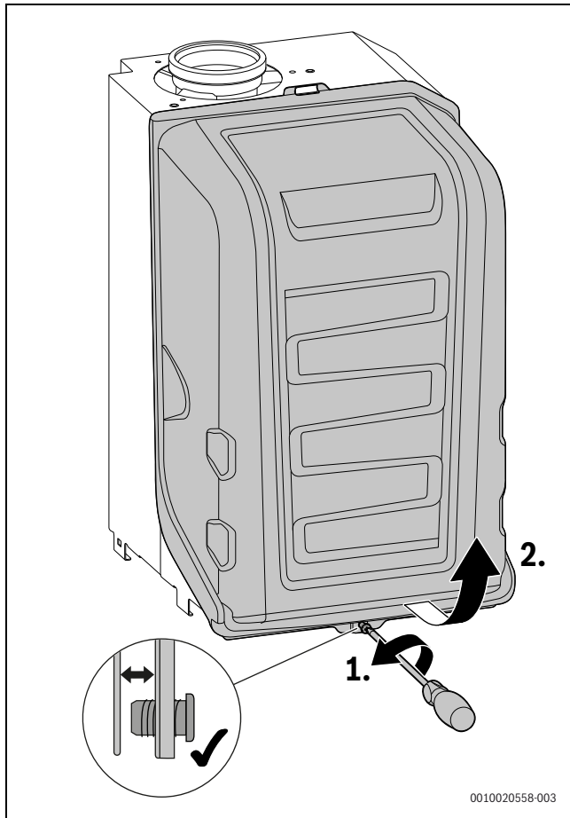
Bild 66 Brennerhaube abnehmen
