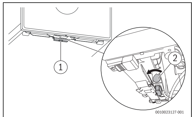
Bild 61 Connect-Key sichern
