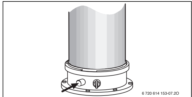
Bild 68 Abgasmessstutzen
