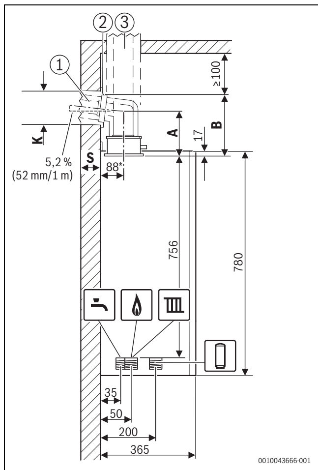
Bild 2 Seitenansicht (mm)
