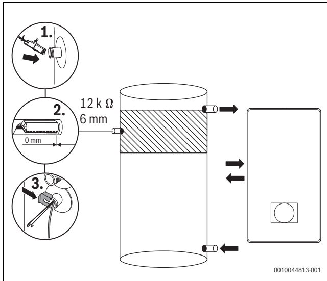
Bild 53 Pufferspeicher-Temperaturfühler 7735502289 einsetzen (bei separatem Warmwasserspeicher und Pufferspeicher)
