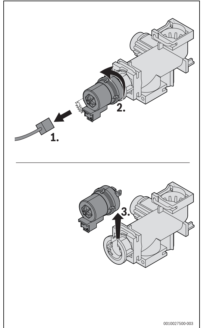
Bild 91 Motor ausbauen (Variante ohne Schrauben)
