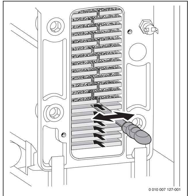
Bild 87 Reinigungsmesser
