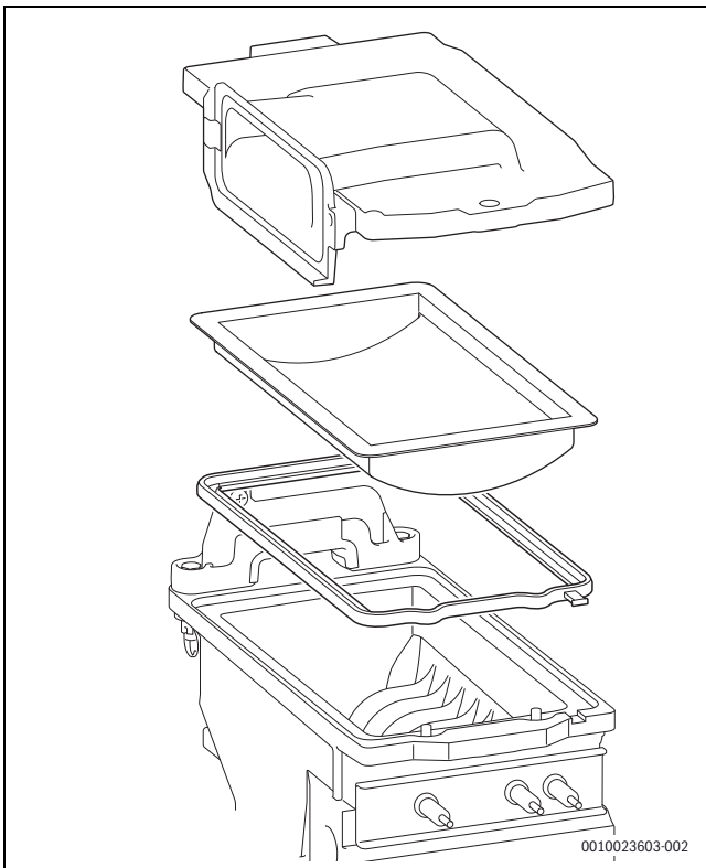
Bild 75 Brenner
