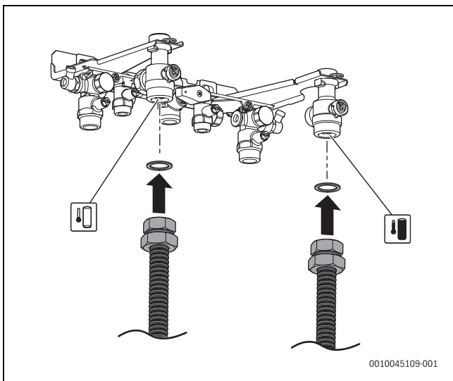
Bild 51 Pufferspeichervorlauf und -rücklauf anschließen
