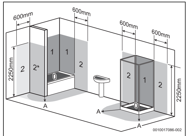
Bild 34 Schutzbereiche (Beispieldarstellung)
