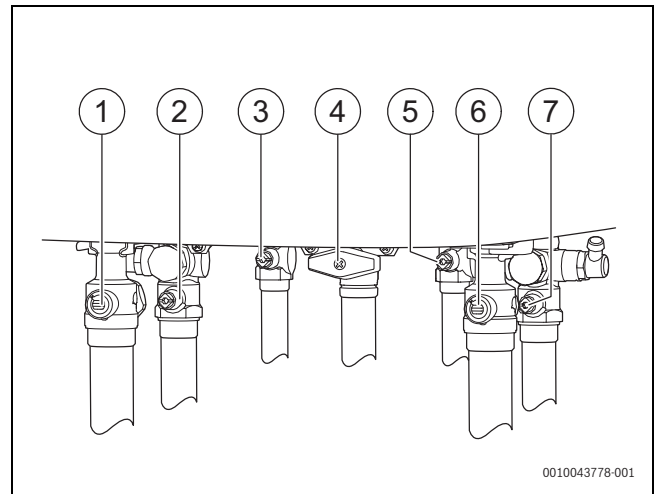
Bild 55 Gas- und wasserseitige Anschlüsse (Zubehör)
