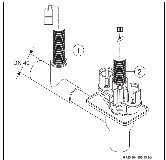
Bild 43 Kondensatschlauch und Schlauch vom Sicherheitsventil am Siphon montieren
