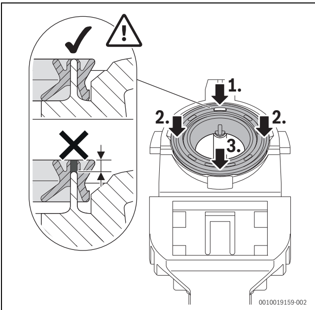
Bild 82 Dichtung andrücken
