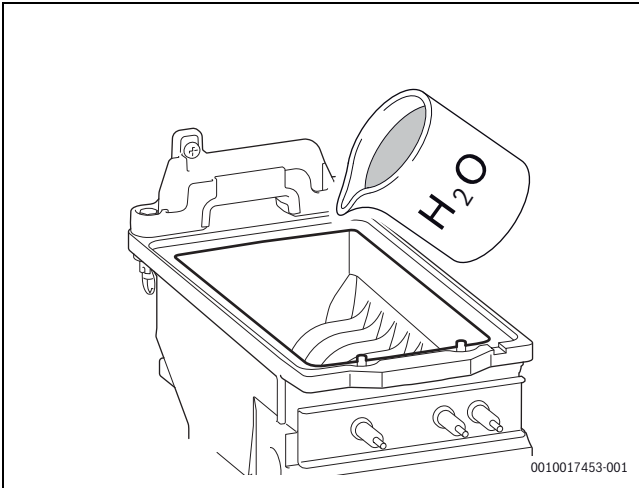
Bild 89 Wärmeblock spülen
