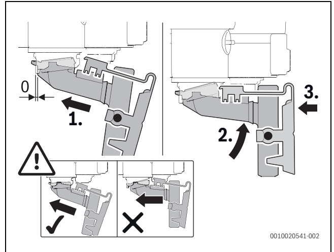
Bild 83 Kondensatsiphon einbauen
