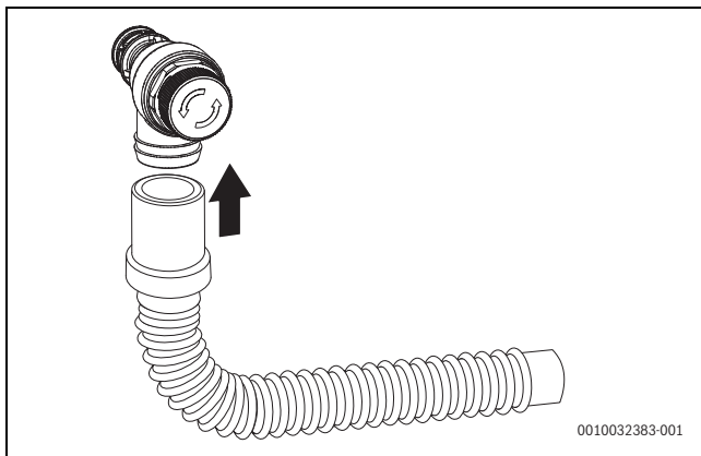
Bild 41 Schlauch am Sicherheitsventil (Heizung) montieren
