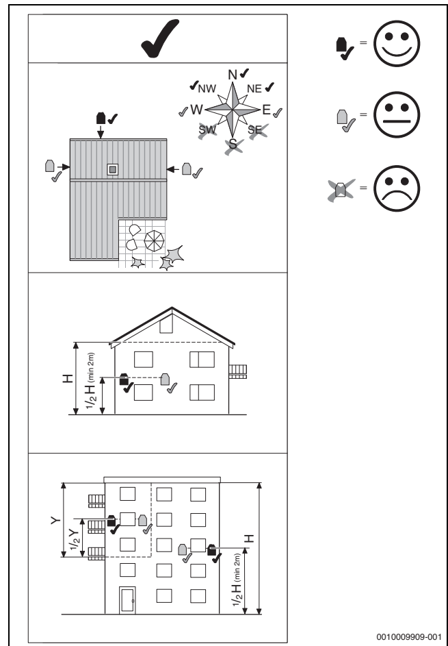
Bild 39 Geeigneter Installationsort des Außentemperaturfühlers
