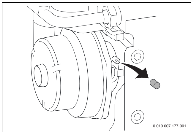
Bild 79 Messstutzen an der Mischeinrichtung
