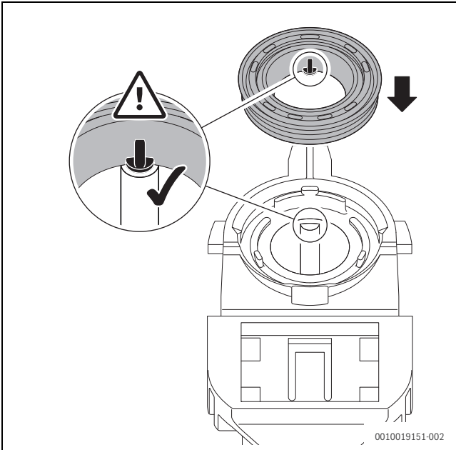
Bild 81 Neue Dichtung am Kondensatsiphon ausrichten
