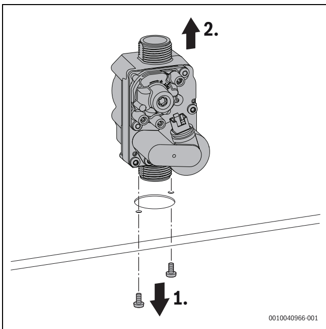
Bild 86 Gasarmatur ausbauen
