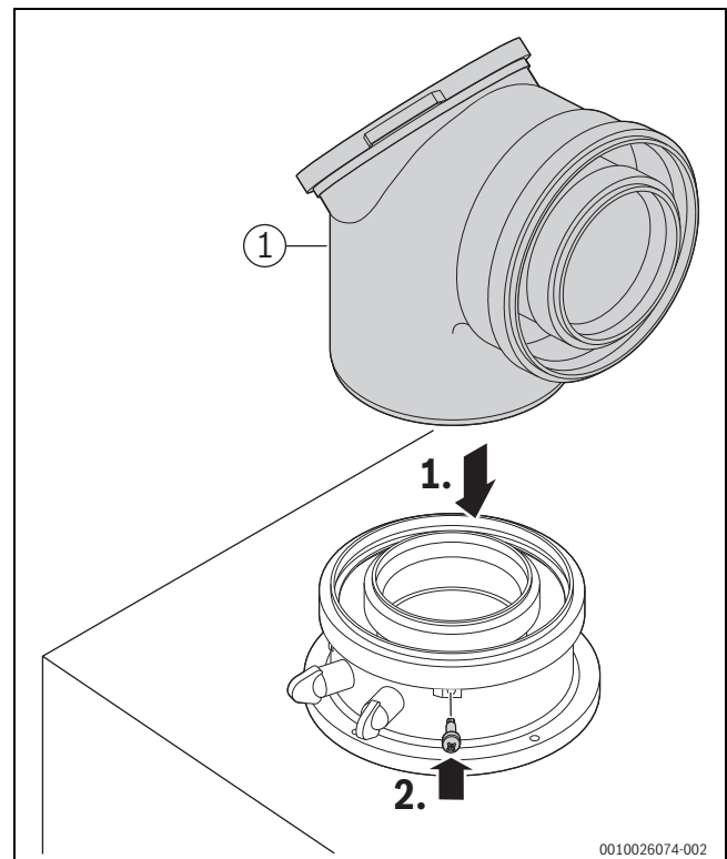
Bild 46 Abgaszubehör einsetzen und mit Schraube sichern
