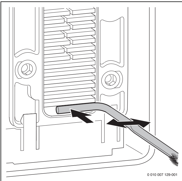
Bild 90 Kondensatwanne reinigen
