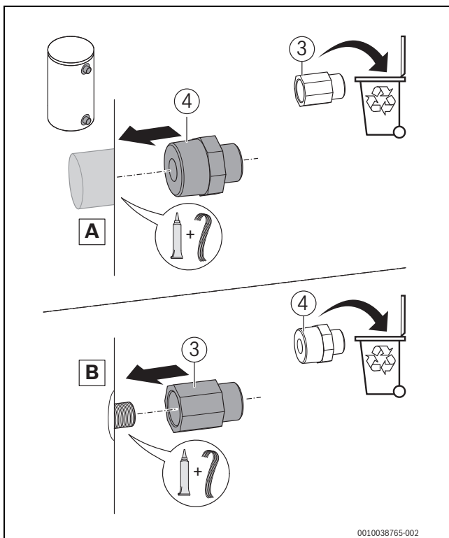
Bild 48 Adapter am oberen und unteren Pufferspeicheranschluss einsetzen
