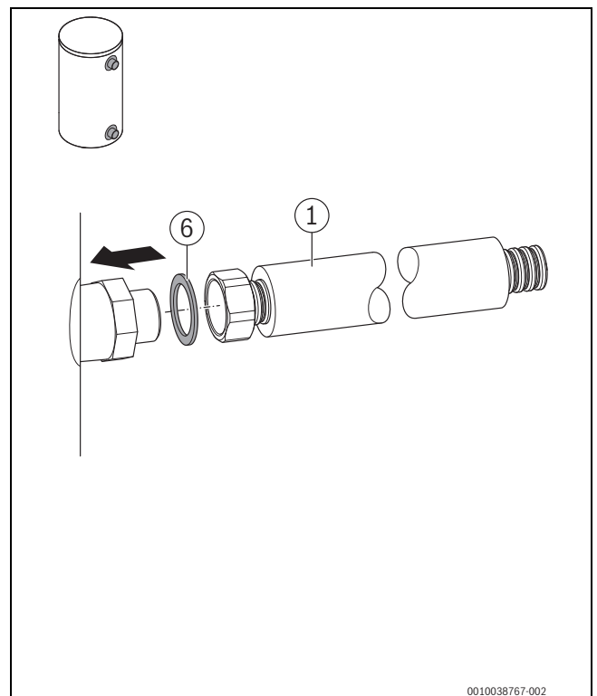
Bild 49 Verbindungsleitungen anschließen
