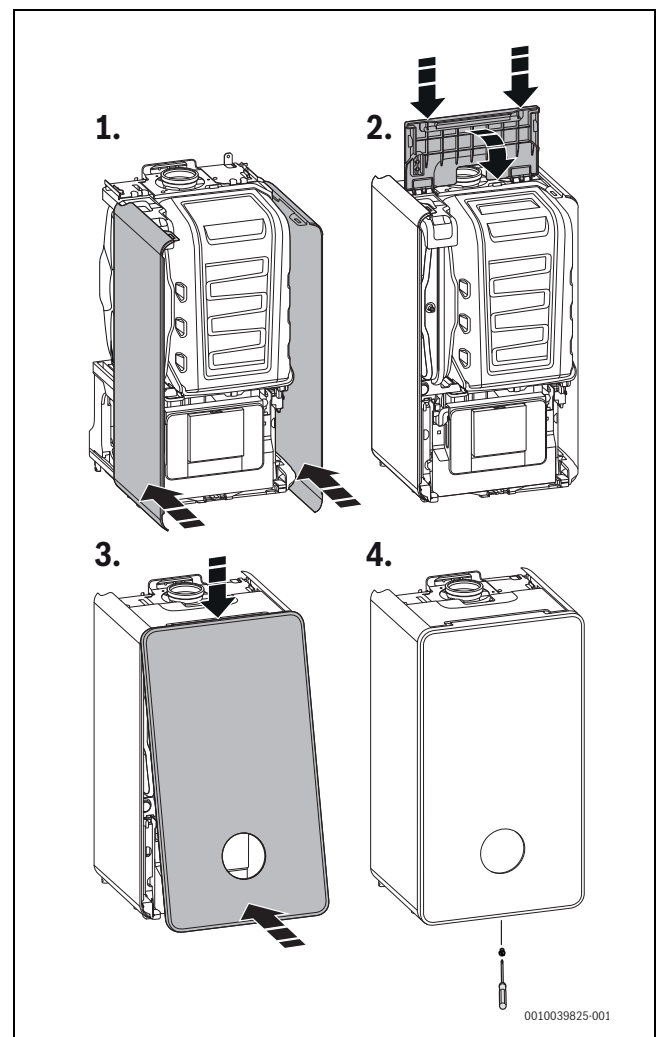
Bild 63 Verkleidung montieren
