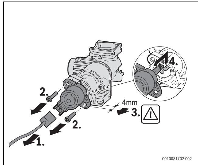
Bild 93 Motor ausbauen (Variante mit Schrauben)
