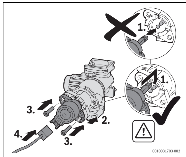
Bild 94 Motor einbauen (Variante mit Schrauben)
