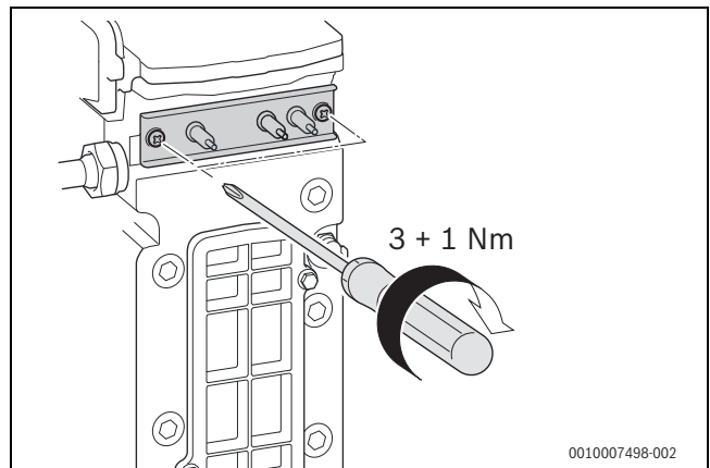
Bild 72 Elektroden-Set montieren
