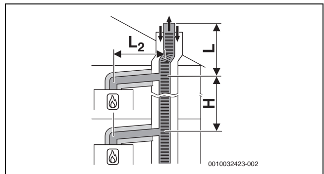
Bild 31 Mehrfachbelegung nach C (14)3x mit kollektiver flexibler Abgasableitung und konzentrischer Luft-Abgas-Führung im Aufstellraum
