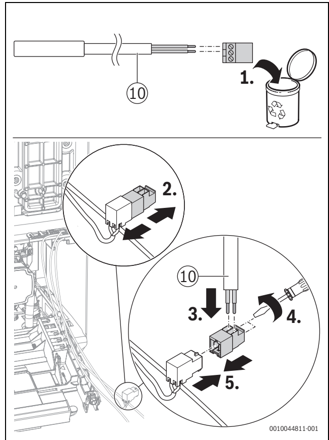
Bild 52 Pufferspeicher-Temperaturfühler anschließen
