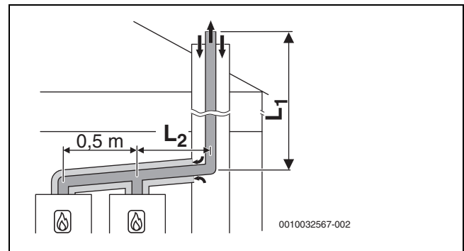
Bild 33 Kaskade mit 2 Geräten: Starre Abgasführung nach C 93x im Schacht und konzentrische Luft-Abgas-Führung im Aufstellraum
