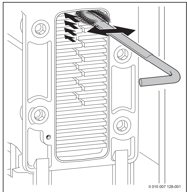
Bild 88 Wärmeblock mit Bürste reinigen
