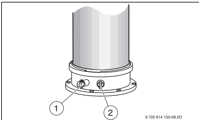
Bild 71 Abgasmessstutzen und Verbrennungsluft-Messstutzen
