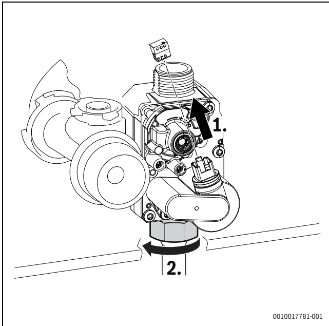
Bild 85 Stecker abziehen und Überwurfmutter lösen
