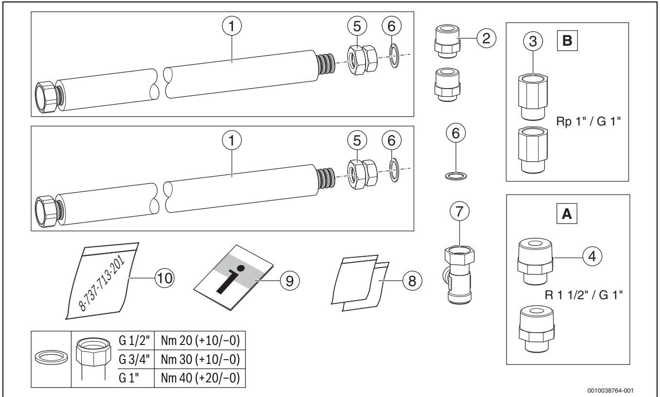
Bild 47 Lieferumfang Zubehör CS39
