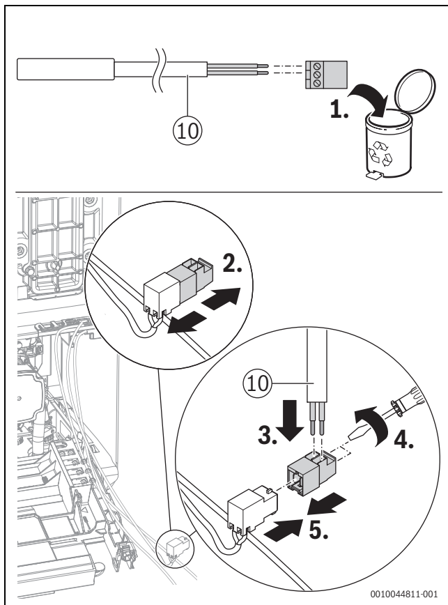
Bild 56 Pufferspeicher-Temperaturfühler anschließen
