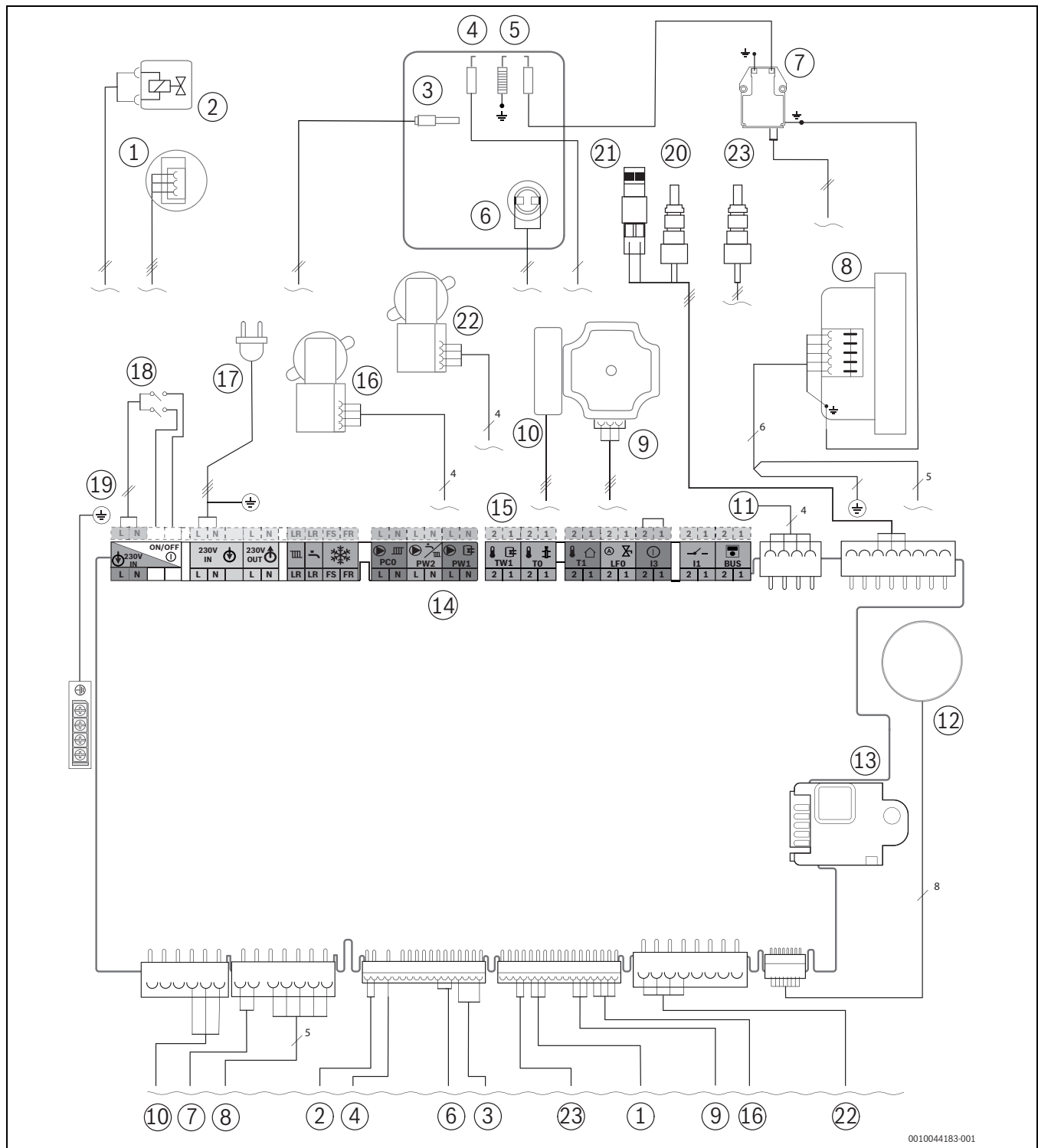
Bild 97 Elektrische Verdrahtung
