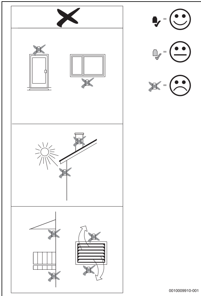
Bild 40 Ungeeigneter Installationsort des Außentemperaturfühlers
