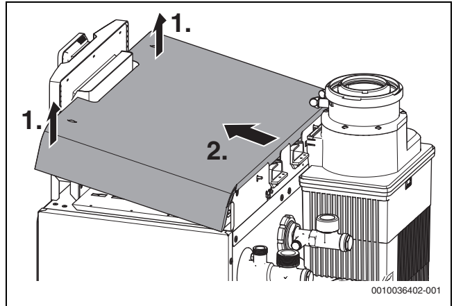
Bild 34 Kesselhaube abnehmen
