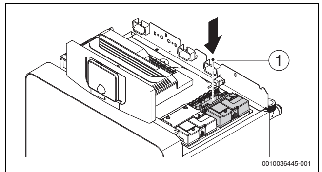
Bild 46 Funktionsmodul verschrauben
