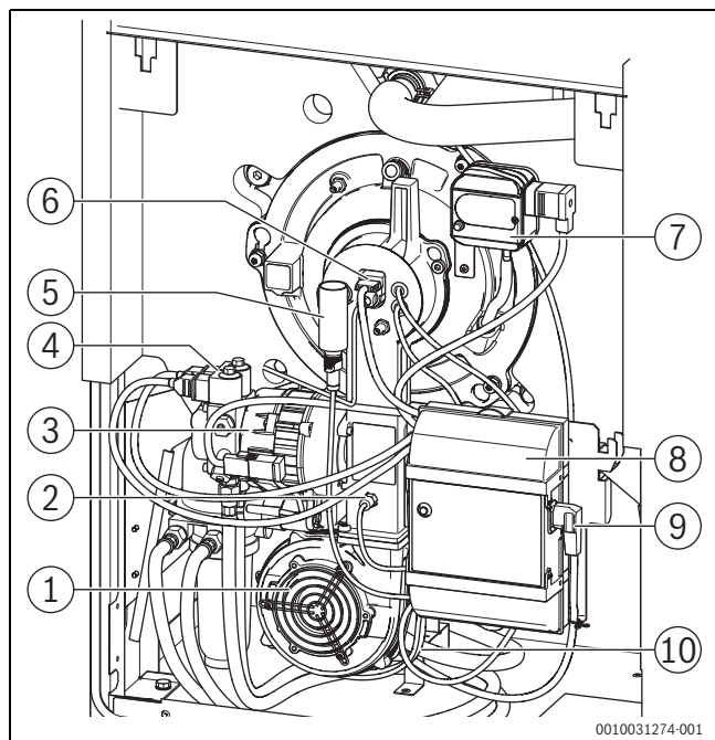
Bild 2 Ölbrenner
