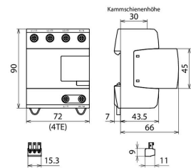
Maßbild DV M2 TNS 255 FM
