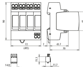
Maßbild DG MP TT ACI 275 FM
