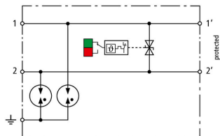
Prinzipschaltbild BCO CL2 BD HC10A 24
