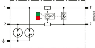
Prinzipschaltbild BCO ML2 BD HF 5
