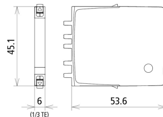
Maßbild BCO MOD ML2 BE 24
