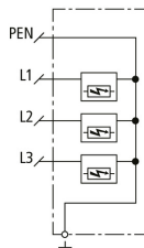
Prinzipialschaltbild DSH ZP 2 TNC 255
