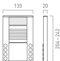
Video-Außenstation Serie AVE
