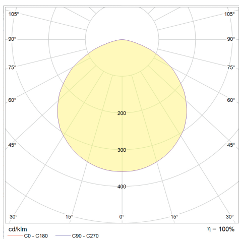
Polardiagramm 840, 120°
