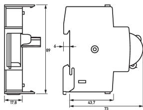
Maßzeichnung Gruppenansicht
