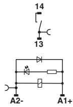
Schaltplan
