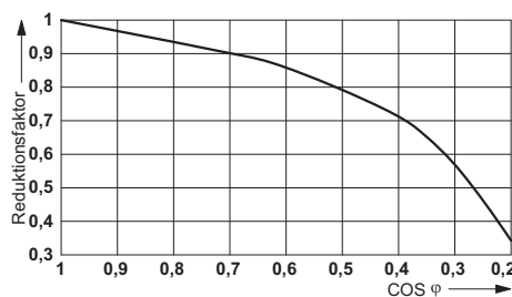
Lebensdauer-Reduktionsfaktor
