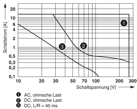
Abschaltleistung
