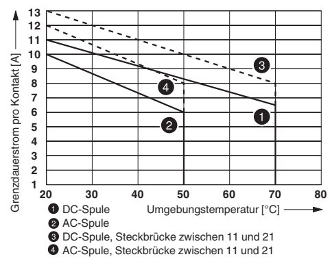
Kontaktderating
