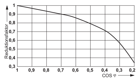
Lebensdauer-Reduktionsfaktor
