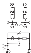
Schaltplan
