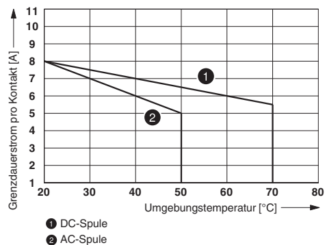
Kontaktderating
