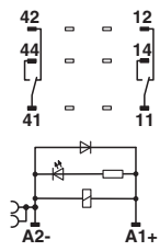
Schaltplan
