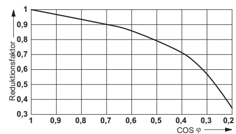
Lebensdauer-Reduktionsfaktor
