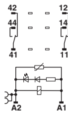
Schaltplan
