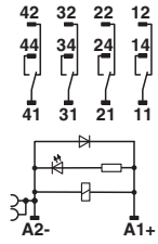
Schaltplan
