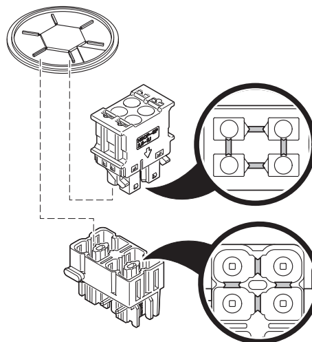
Schemazeichnung
