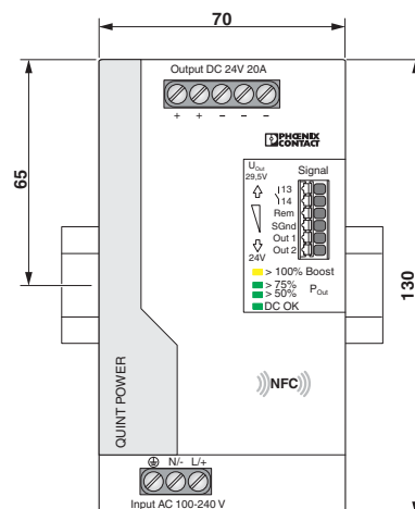
Maßzeichnung
