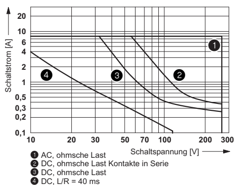
Abschaltleistung
