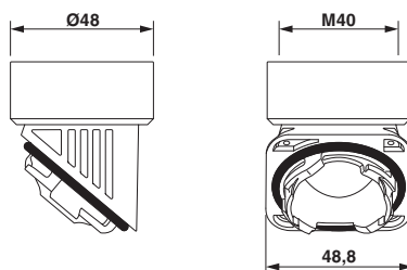
Maßzeichnung
