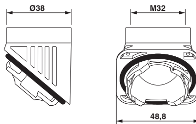
Maßzeichnung
