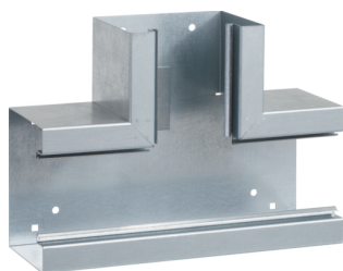
T-Stück aus Grundprofil zu BRS 100x130mm Oberteil 80mm aus Stahlblech verzinkt
