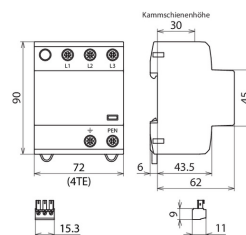
Maßbild DSH B TNC 255 FM
