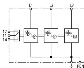
Prinzipschaltbild DSH B TNC 255 FM
