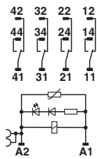
Schaltplan
