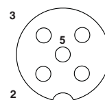
Polbild Buchse M12, 5-polig, A-kodiert, Ansicht Buchsenseite
