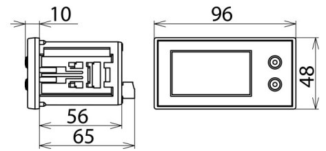
Maßbild DPAN L
