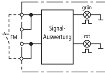
Prinzipschaltbild DPAN L
