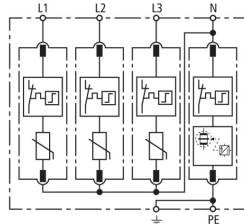
Prinzipschaltbild DG M H TT 275
