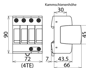
Maßbild DG M H TT 275
