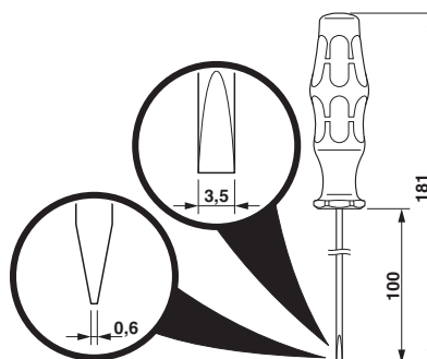
Maßzeichnung
