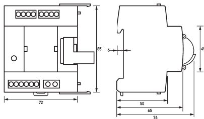
Maßzeichnung Gruppenansicht
