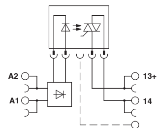
Schaltplan
