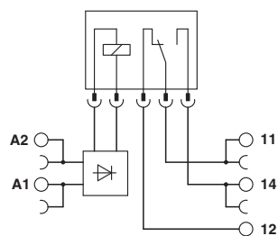
Schaltplan
