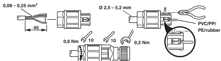
Funktionszeichnung
