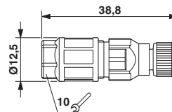
Maßzeichnung
