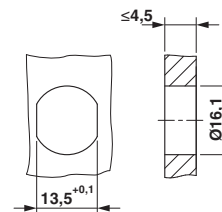
Gehäuseausschnitt für M16-Befestigungsgewinde, Montagewand mit Durchgangsbohrung (alternativ mit Fläche als Verdreherschutz für Montagewandstärken >2 mm bis max. 4,5 mm)
