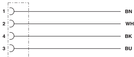
Schaltplan
