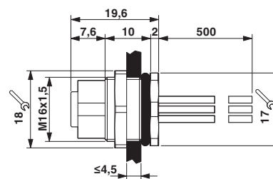
Maßzeichnung
