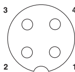
Polbild Buchse M12, 4-polig, A-kodiert, Ansicht Buchsenseite
