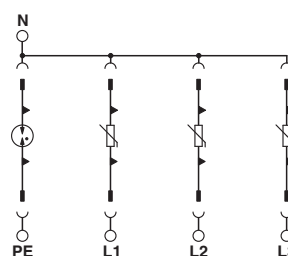
Schaltplan
