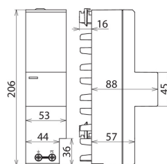
Maßbild DSH ZP B TT 255
