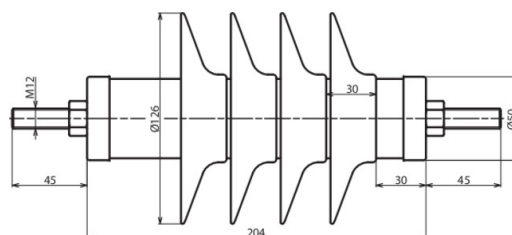
Maßbild DMI 21 10 1 H
