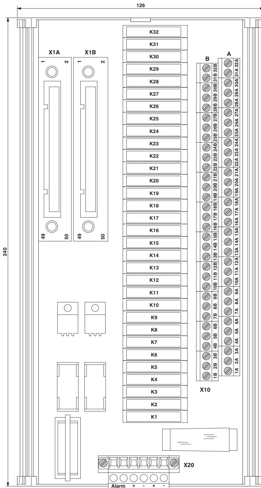
Maßzeichnung
