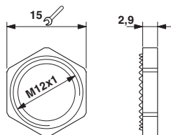
Maßzeichnung
