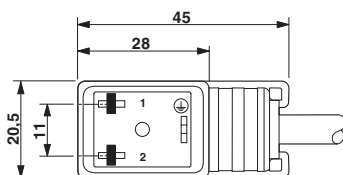
Ventilstecker, Bauform BI
