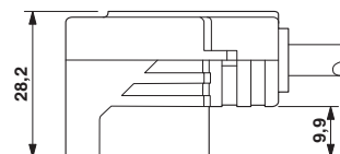
Ventilstecker, Bauform A, Seitenansicht
